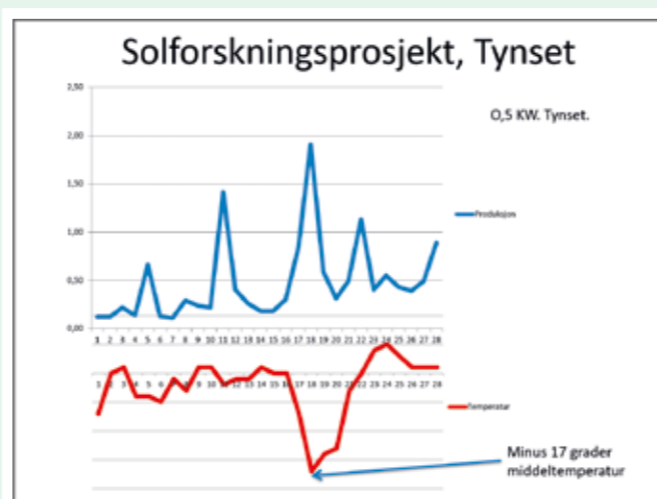
Sammenheng mellom temperatur og strømproduksjon. Klart og kaldt vær med mye sol gir høy produksjon
